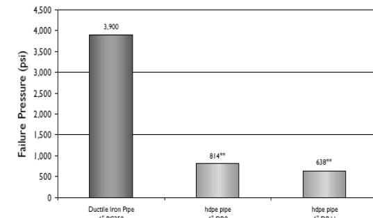
شکل ۴. مقایسه مقاومت در برابر فشار هیدرواستاتیک لوله پلی اتیلن سنگین و چدن نشکن
