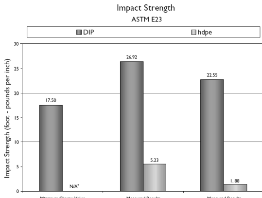
شکل ۵. مقایسه استحکام در برابر ضربه لوله پلی اتیلن سنگین و چدن نشکن
